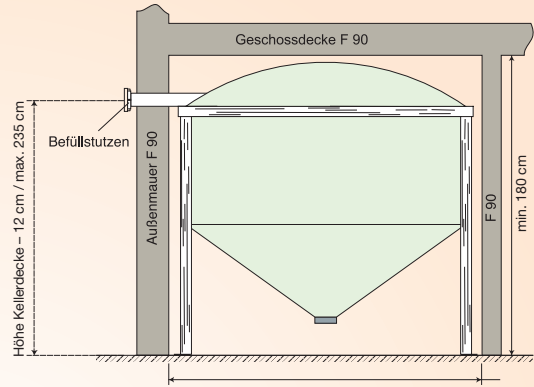
Abb. 32: Querschnitt eines Heizraums mit Gewebesilo
